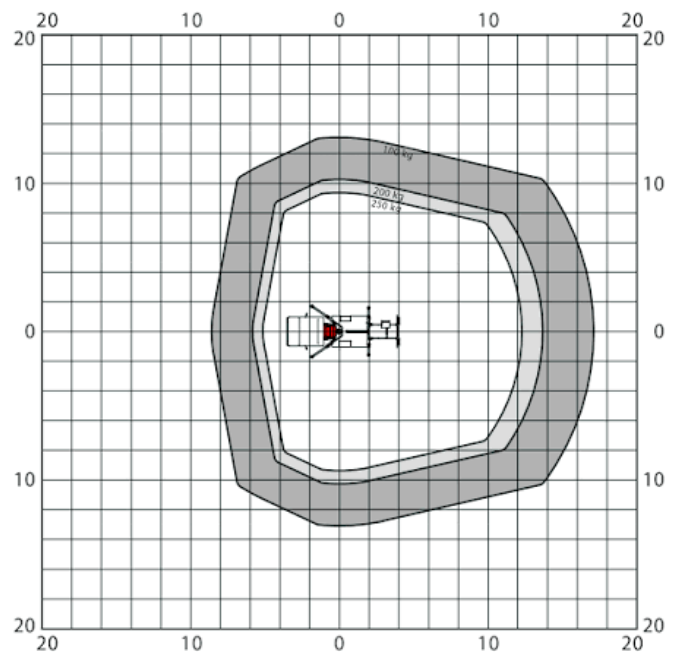
Arbeitsbereich - Draufsicht
