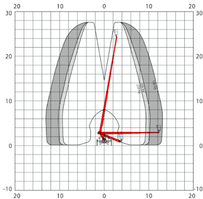
Arbeitsbereich - Seitenansicht
